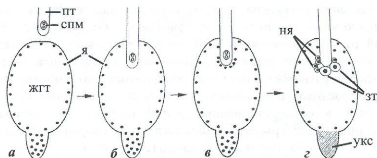
Рис. 4.2. Схема двойного оплодотворения у гнетума.
