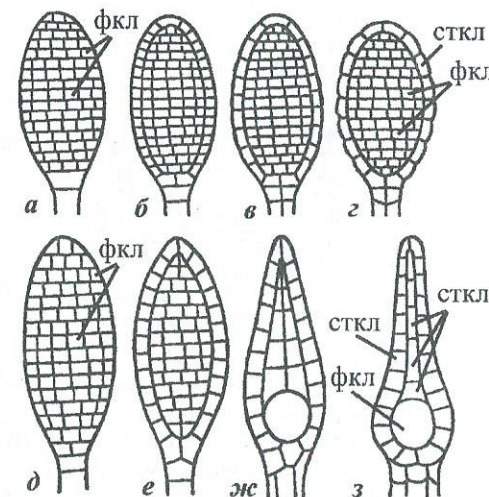
Рис. 1.11. Происхождение антеридиев (а–г) и архегониев (д–з) растений из многоклеточных гаметангиев водорослей.
