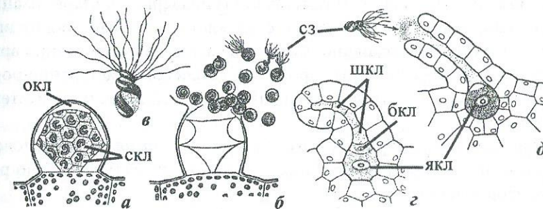
Рис. 1.10. Гаметангии папоротника щитовника мужского.
