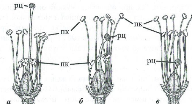
Рис. 2.43. Гетеростилия у дербенника иволистного.
