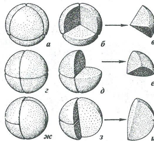
Рис. 1.3. Основные типы тетрад спор (а, г, ж) и расположение в них трилетних (б, в) и монолетных (д, е, з, и) спор.
