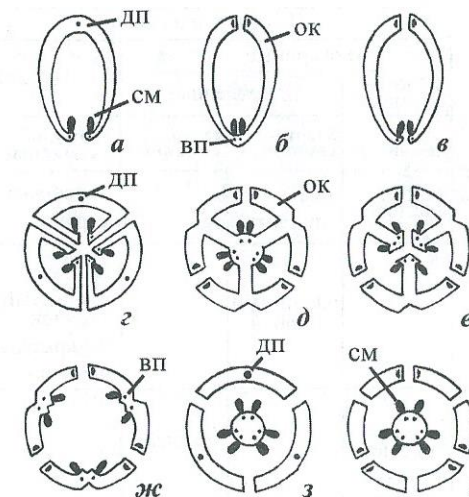
Рис. 2.54. Некоторые способы вскрывания плодов.
