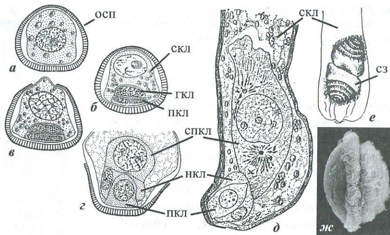
Рис. 2.5. Мужской гаметофит сфагновых.
